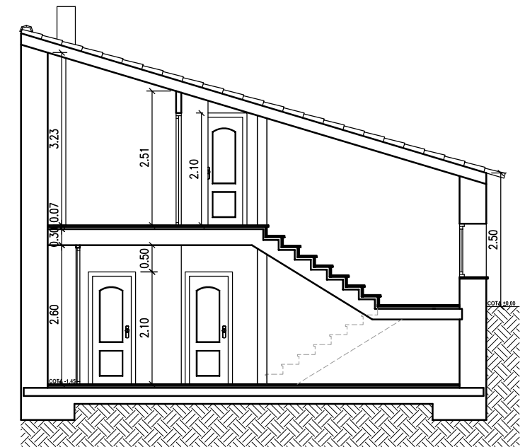
SECCIÓN B-B'
