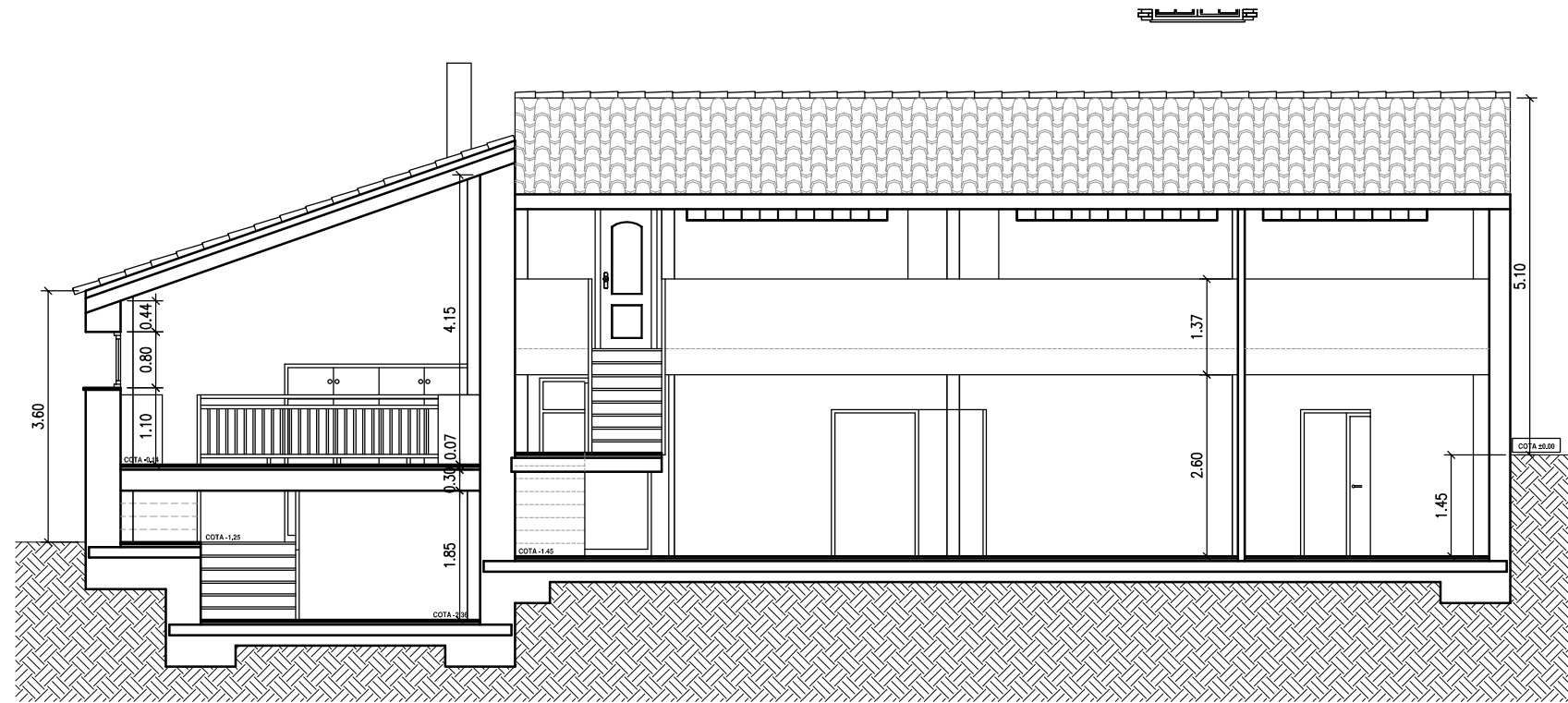
SECCIÓN A-A'
